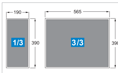
Mit standardisiertem Schubladen-Innenmaß passend für MATADOR MTS-Moduleinlagen.
